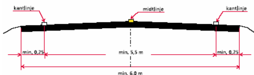
Figur 1 Breddkrav för utmärkning av midtlinje. Statens vegvesen, 2001, s. 23.
